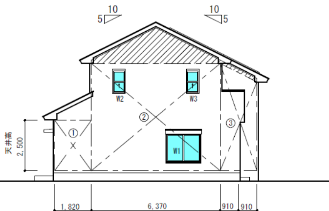
西側立面図
