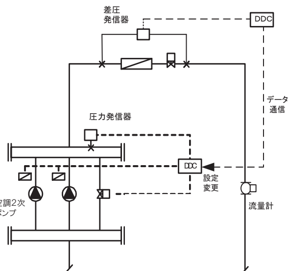
事例1:事業No.103/106/109 空調2次ポンプの末端差圧制御
