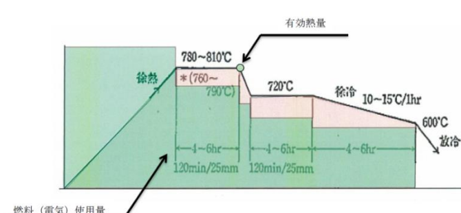
図.3 軸受鋼の焼きなまし曲線/燃料(電気)投入パターン例
