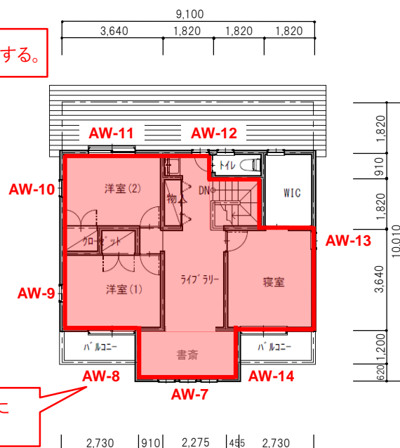
2階平面図
