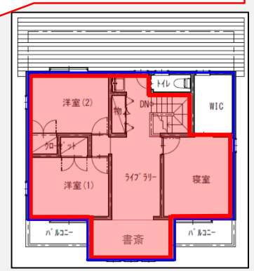
2階平面図
