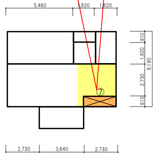
2階床求積図
