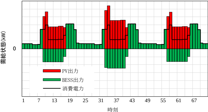
両地区による需給運用計画
