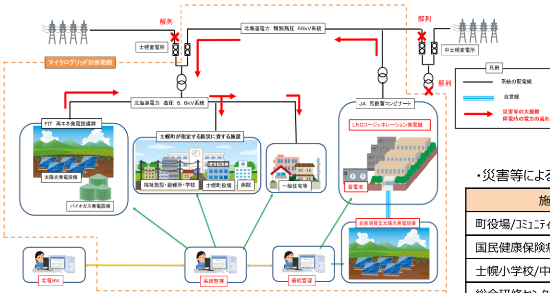
土幌町マイクログリッド 概要図
