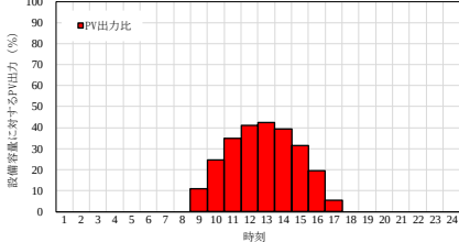
※発電カーブは推計値 太陽光発電出力割合（冬季）
