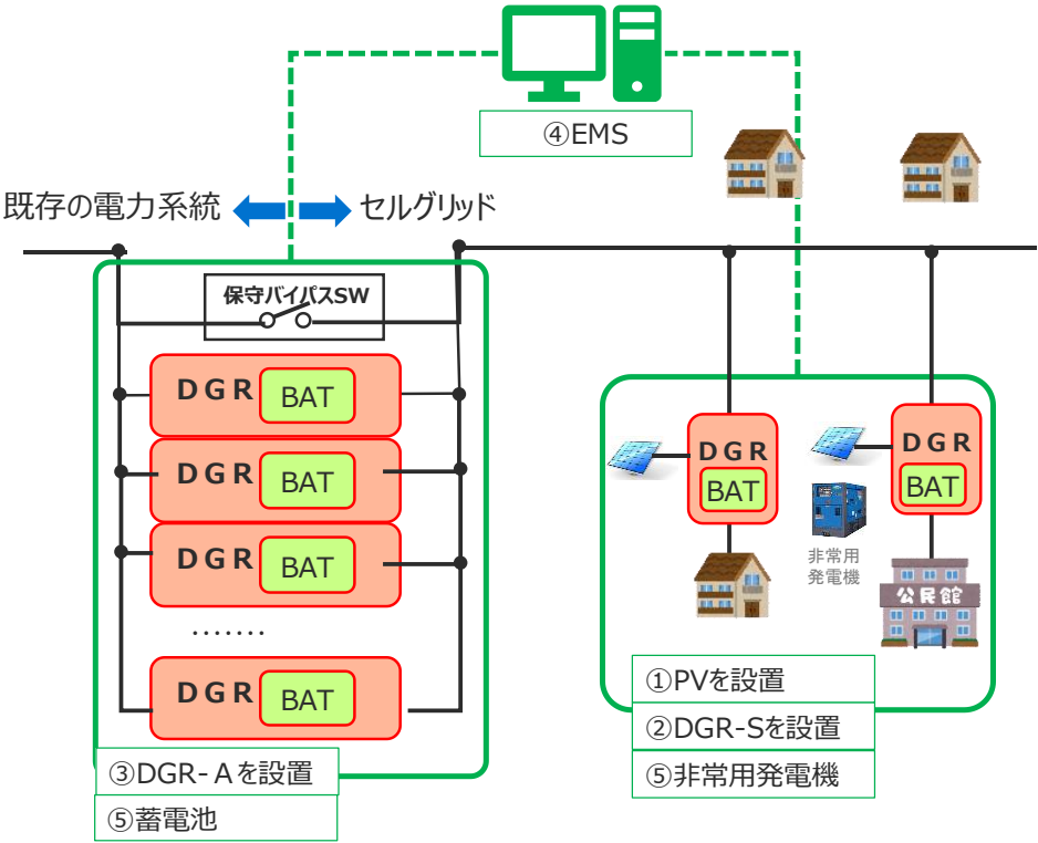
・マイクログリッドを構成する設備の概要案：
