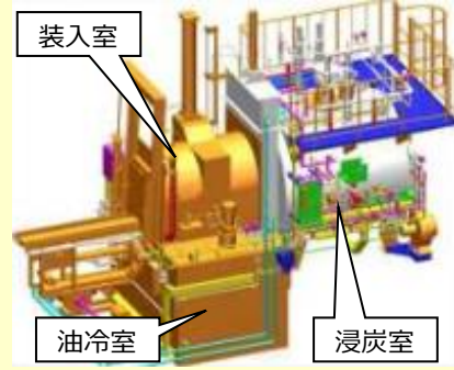
ガス浸炭設備
