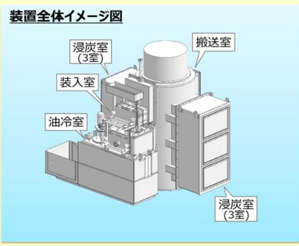
真空浸炭設備
