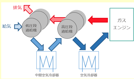
図1 2段過給システム図
