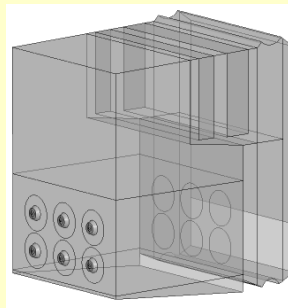
二胴水管前焚ボイラ (F型)
