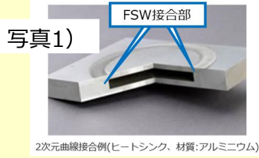
2次元曲線接合例(ヒートシンク、材質:アルミニウム)
