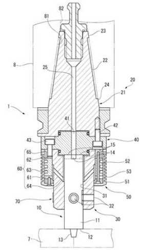
図1) 特許第6787764号付図
