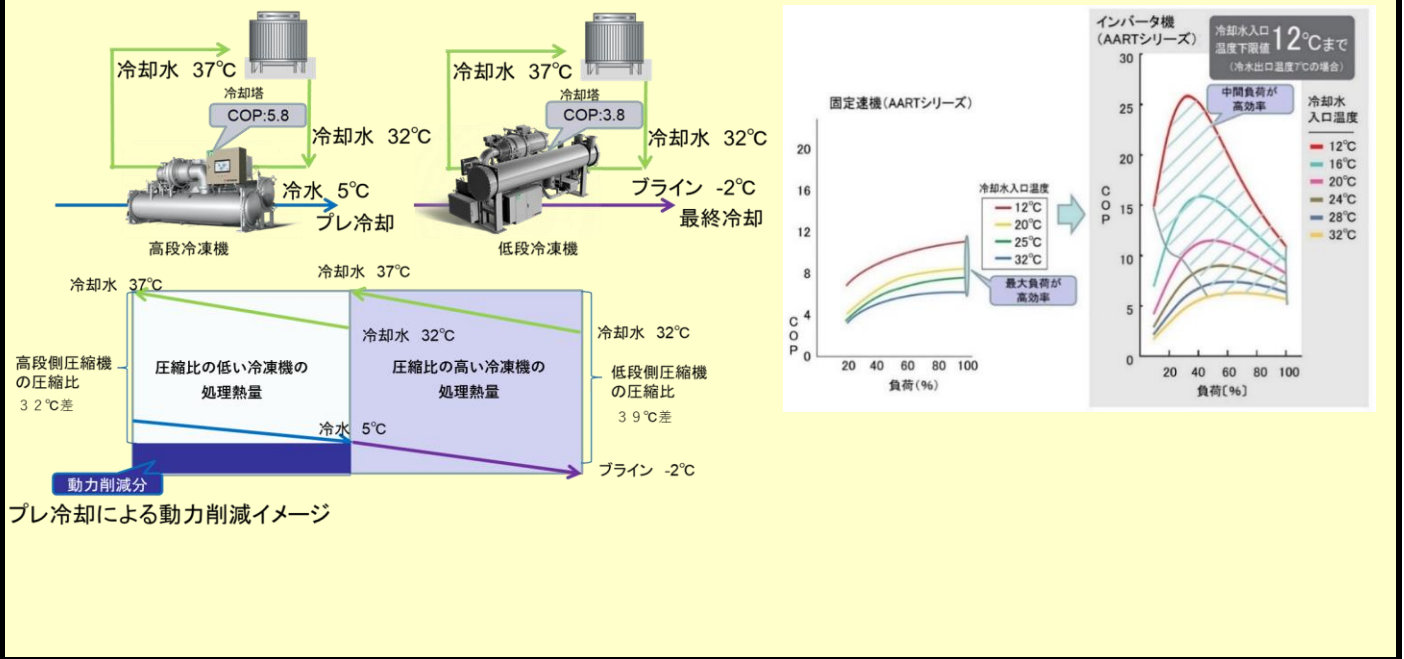
図ー1 プレ冷却による動力削減イメージ、
