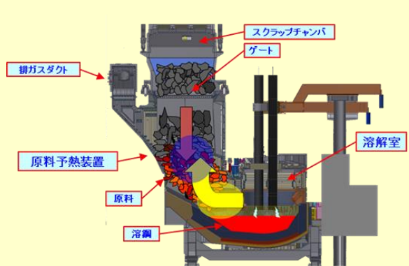
図2 ECOARC-FIT概念図
