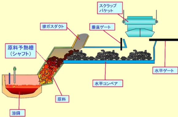
図1 ECOARCTM、ECOARC-light概念図
