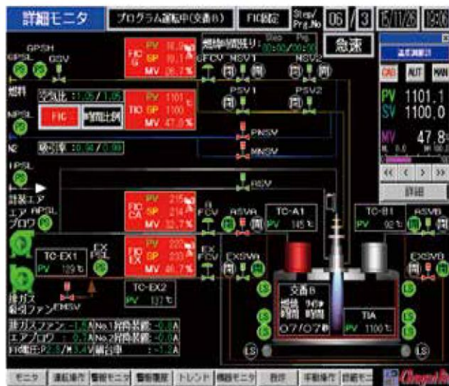
タンディッシュ予熱最適燃焼システム
