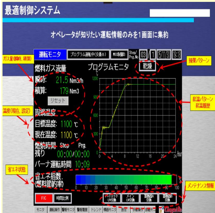
タンディッシュ予熱最適燃焼システム
