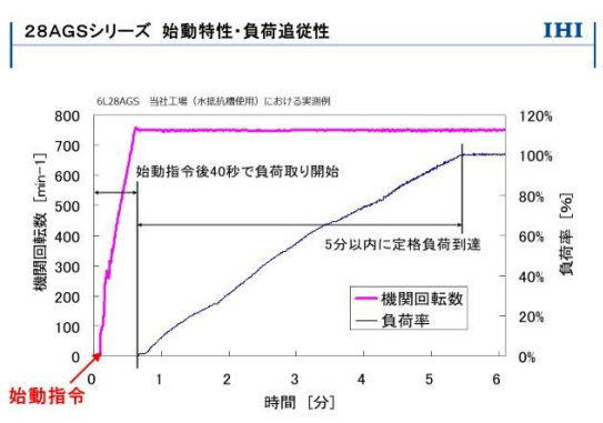
図3 始動時間・負荷追従性
