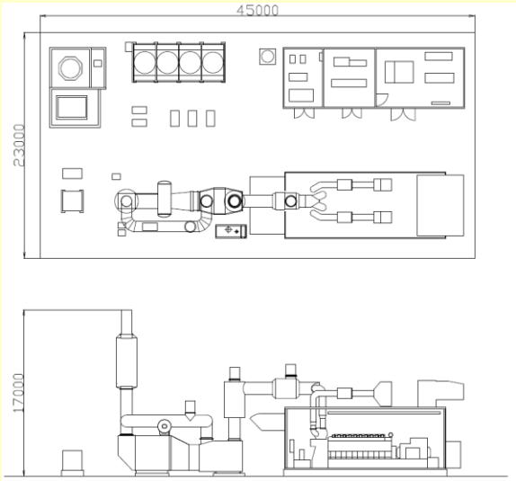
図2 配置図 (W20V31SG)
