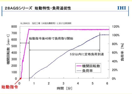
図3 始動時間・負荷追従性
