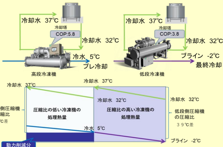
プレ冷却による動力削減イメージ
