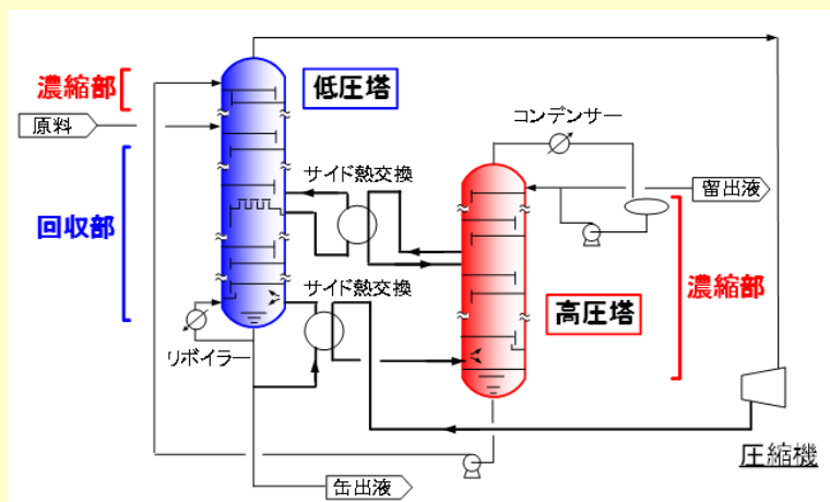
図1 SUPERHIDIC®装置システム
