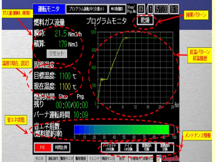
タンディッシュ予熱最適燃焼システム
