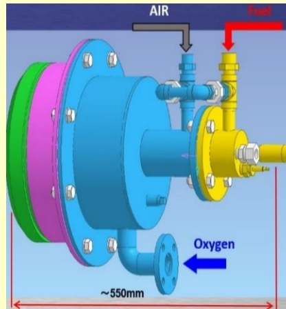
タンディッシュ予熱専用拡散燃焼式酸素バーナ
