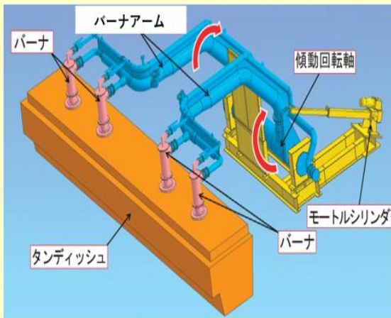
タンディッシュ予熱装置構成
