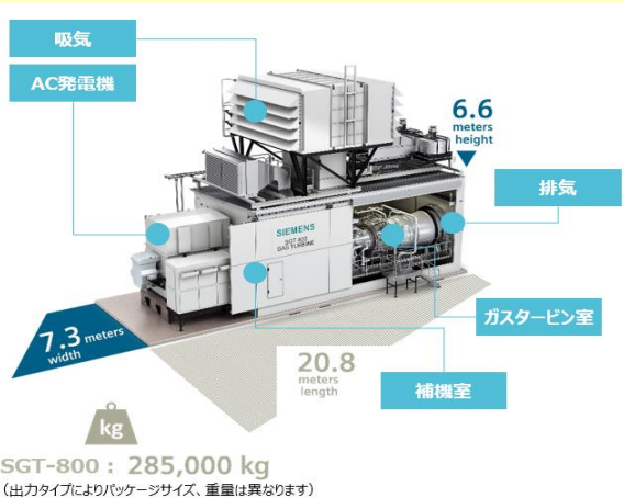
SGT-800外形図
