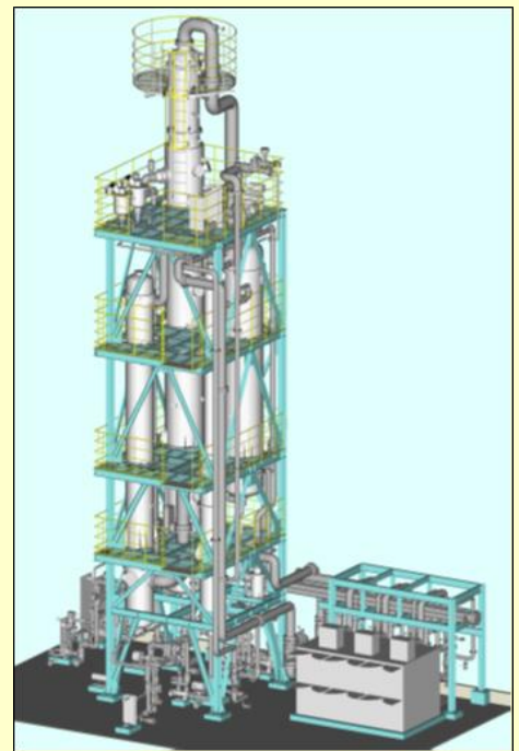
ヒートポンプ式アンモニア回収装置 3Dイメージ図
