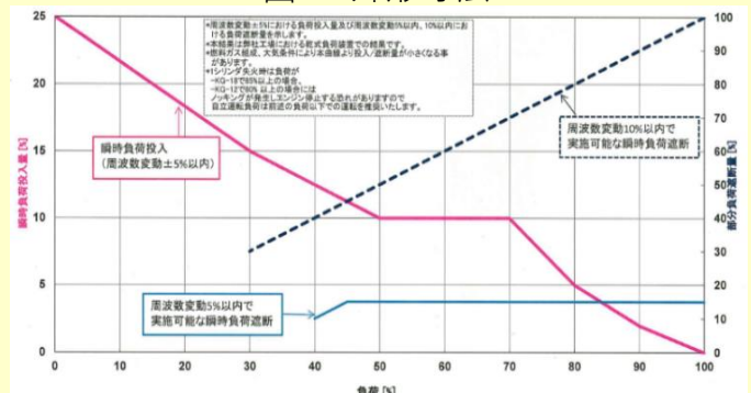
図4 瞬時負荷投入/遮断曲線 (KG-18-V (オプション))
