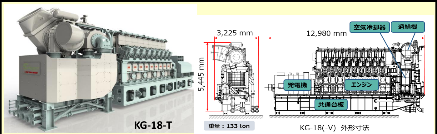
図1 ガスエンジン外観
