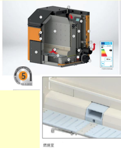
燃焼室
