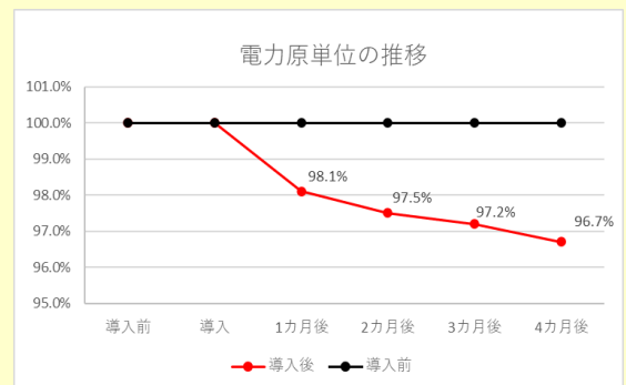
図3 ターンコイル導入例
