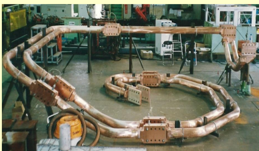
図1 ターンコイル（陽極側導体）
