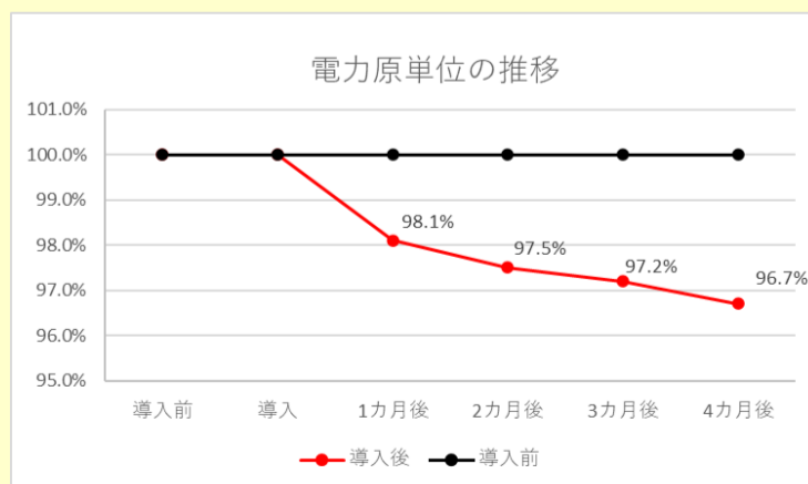
図3 ターンコイル導入例
