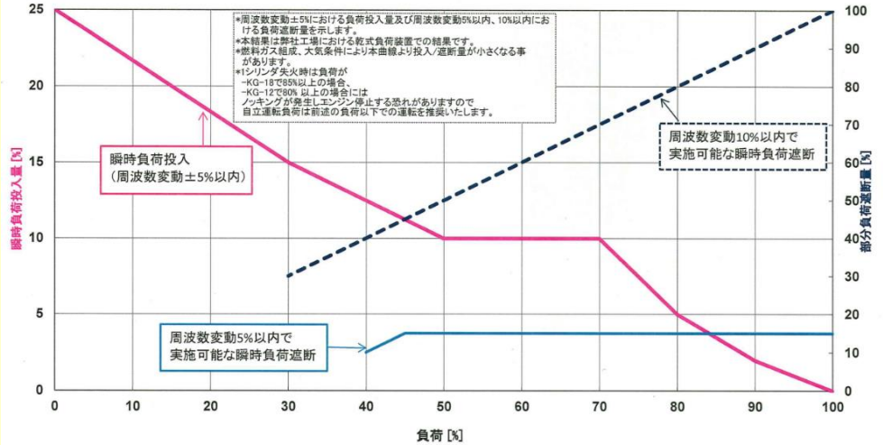
図4 瞬時負荷投入/遮断曲線
