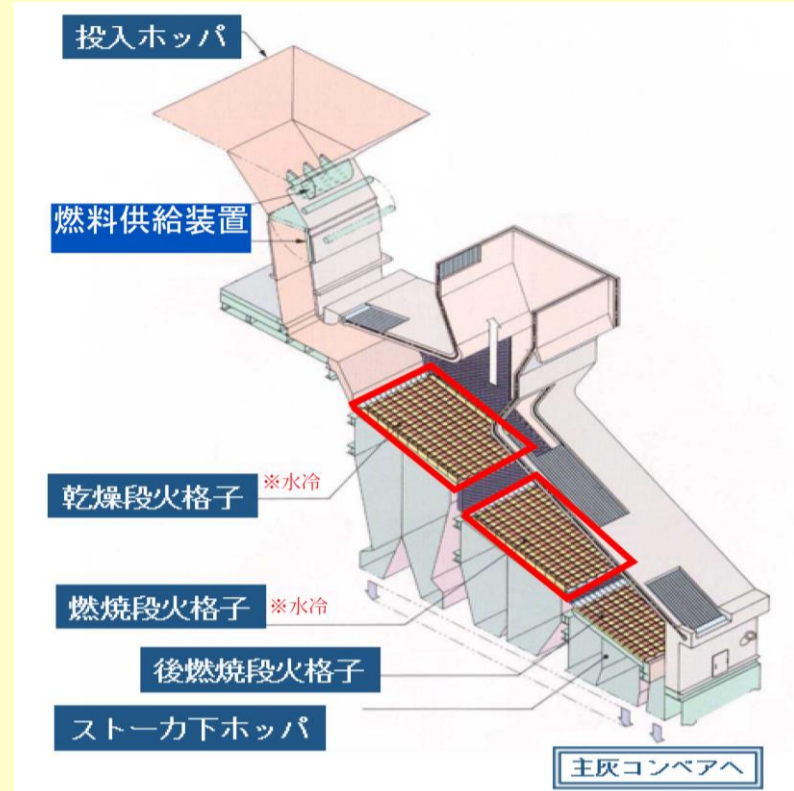
燃焼室模式図
