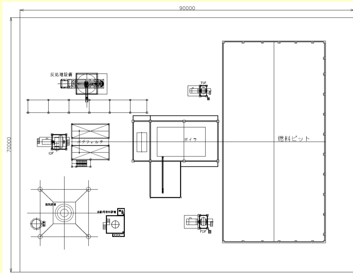
プラント全体図
