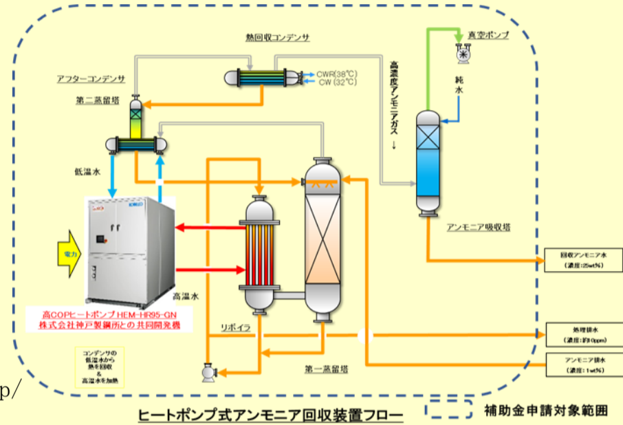
ヒートポンプ式アンモニア回収装置フロー 補助金申請対象範囲
