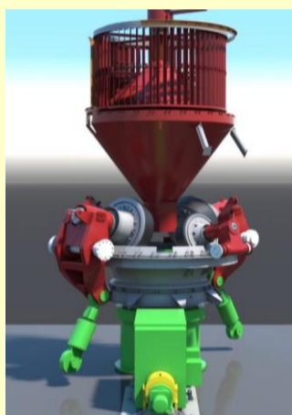
縦型ミルの構造
