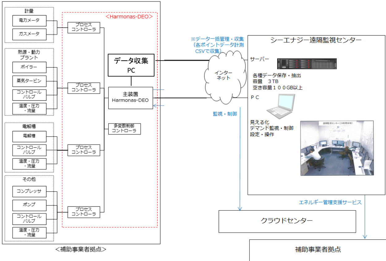
システム・機器構成図
