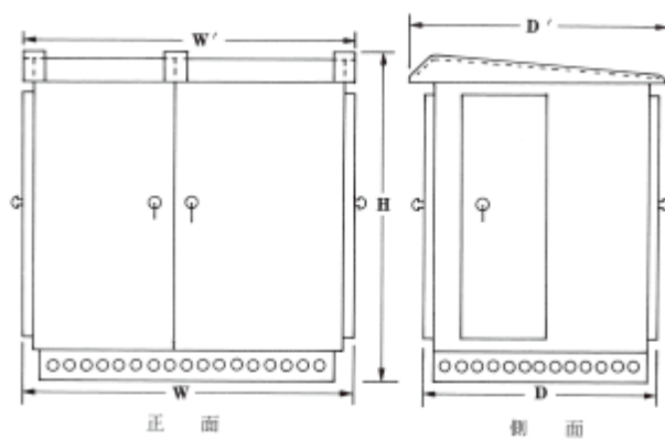
図 - 8 外形寸法
