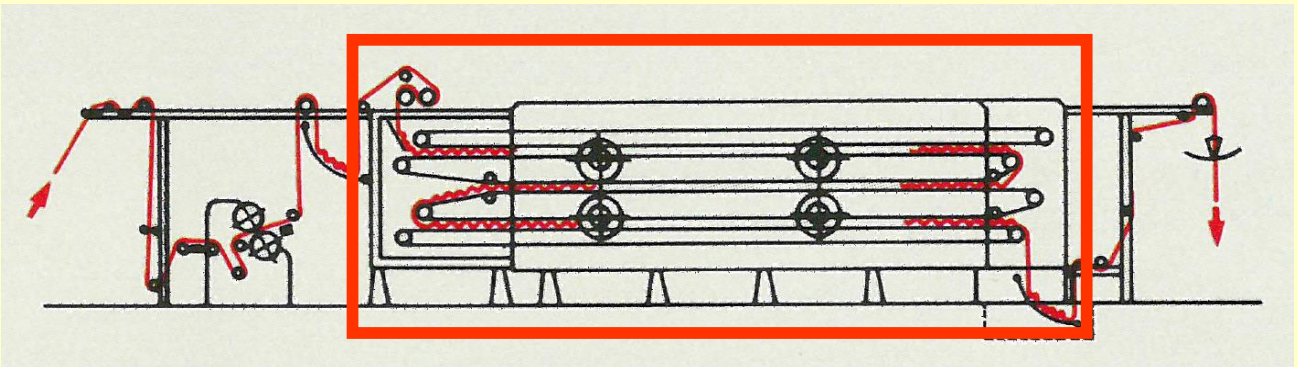
エネルギー負荷設備は赤枠内の設備と煙道・分割型SUSプレート式熱交換器です。 前後は付帯設備（入口装置・パディングマングル・出口振り落とし装置など）です。
