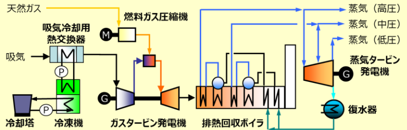
蒸気タービンコンバインド型コージェネレーションシステム
