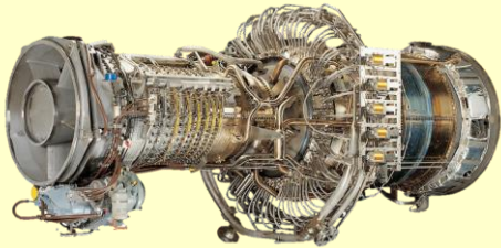
LM2500+G4ガスタービン
