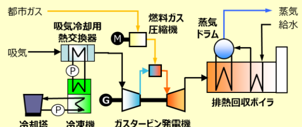
単純コージェネレーション
