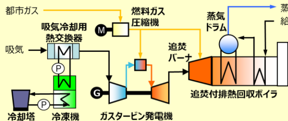
追焚付排熱回収ボイラコージェネレーション
