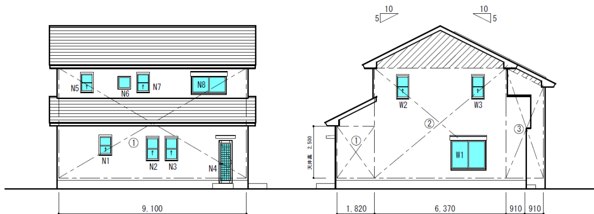
北側立面図
